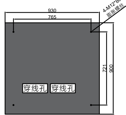
水泥基础俯视图
