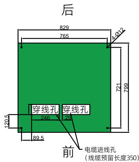
480kW直流桩 外壳底座俯视图 (自上向下看)
