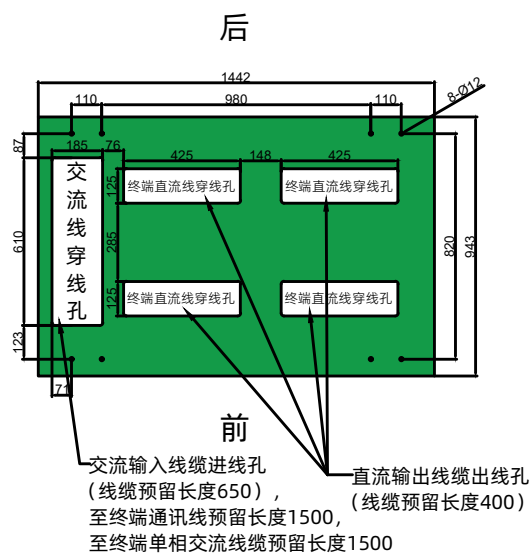
480~720kW 充电堆 外壳底座俯视图 (自上向下看)
