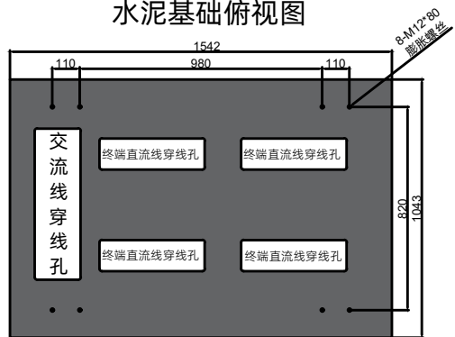
水泥基础视图
