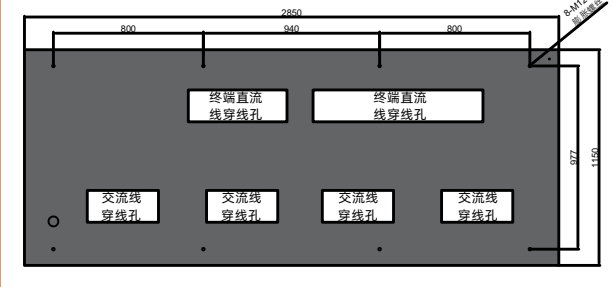
水泥基础俯视图
