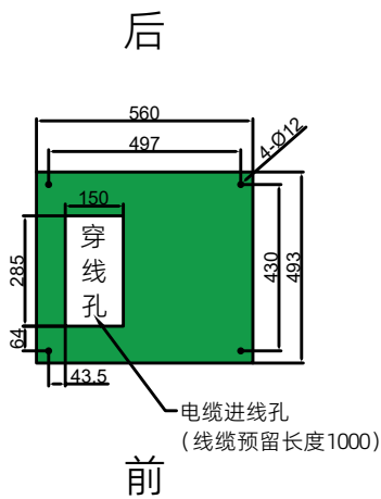
液冷终端机- 400A- 600A- 800A 外壳底座俯视图 (自上向下看)
