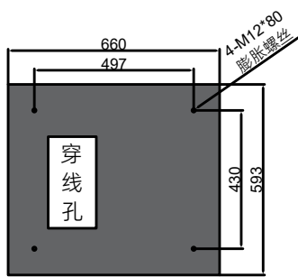
水泥基础俯视图
