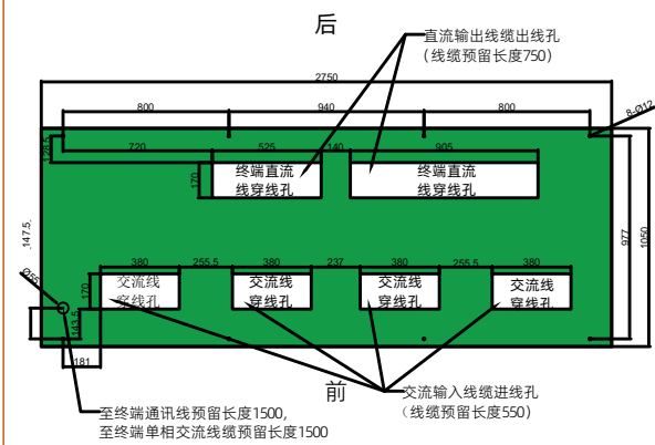
1440~2560kW 充电堆 外壳底座俯视图 (自上向下看)
